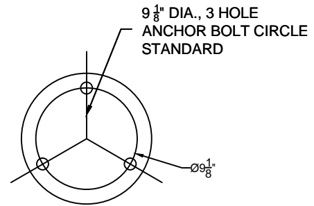
BOLT CIRCLE SCALE: 1" = 1'-0"
