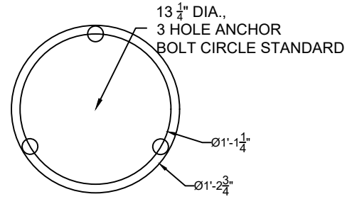
BOLT CIRCLE 2 SCALE: 1" = 1'-0"
