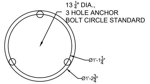
BOLT CIRCLE SCALE: 1" = 1'-0" 2
