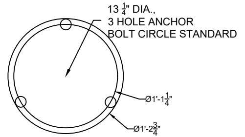
BOLT CIRCLE SCALE: 1" = 1'-0"
