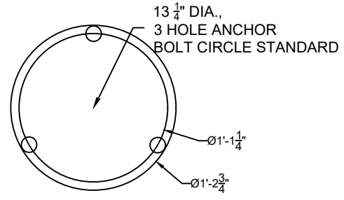
BOLT CIRCLE 2 SCALE: 1" = 1'-0"
