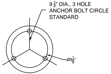
BOLT CIRCLE SCALE: 1" = 1'-0"
