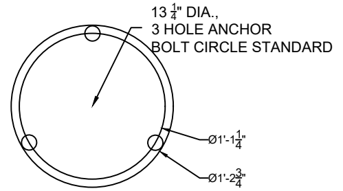
BOLT CIRCLE SCALE: 1" = 1'-0"
