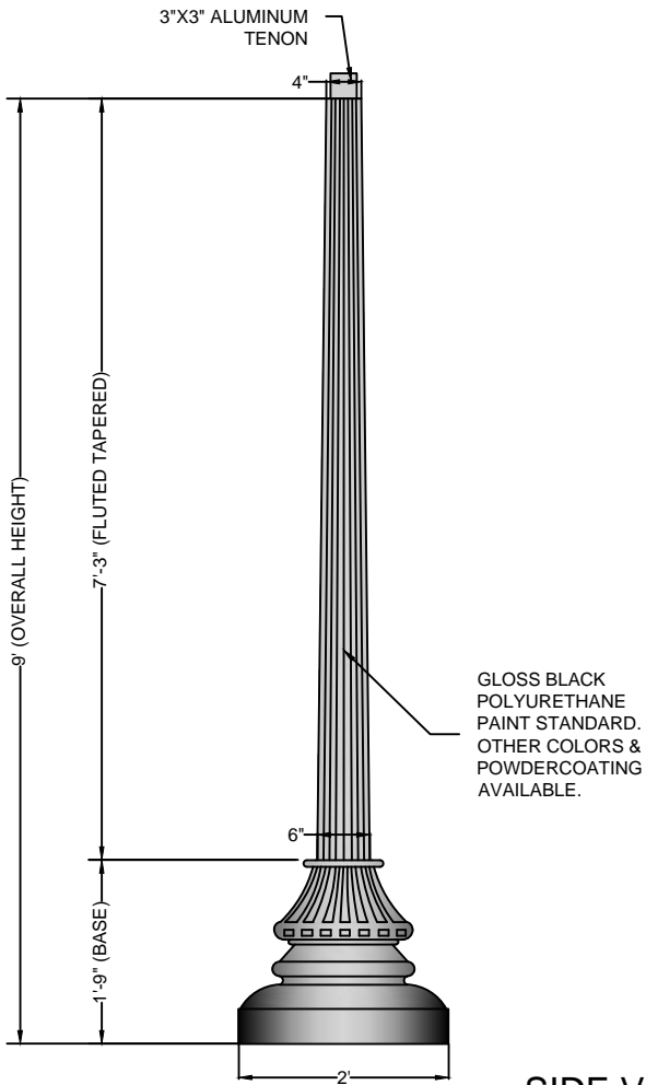
SIDE VIEW SCALE: 1/2" = 1'-0" 1
