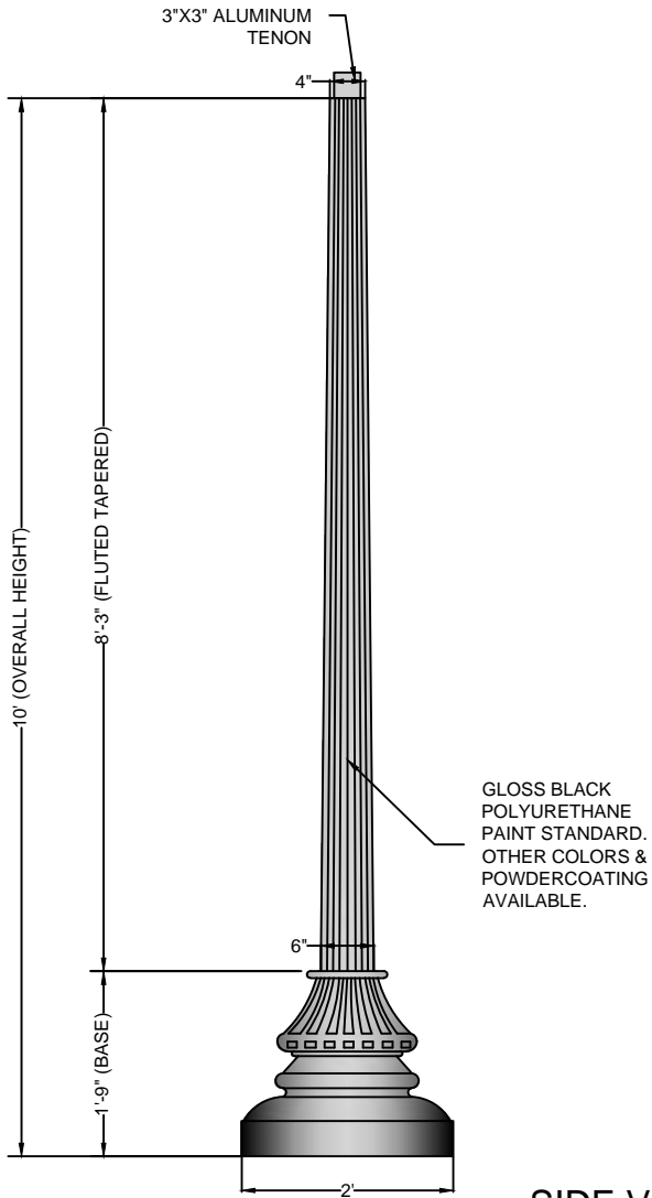
SIDE VIEW SCALE: 1/2" = 1'-0" 1
