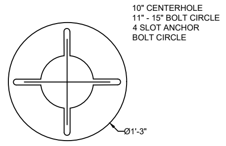
BOLT CIRCLE 2 SCALE: 1" = 1'-0"
