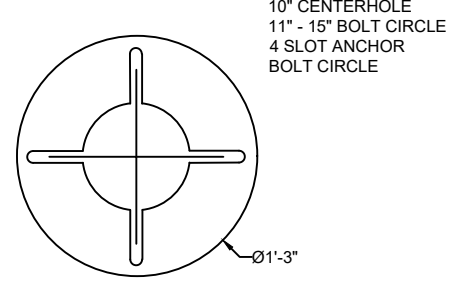
BOLT CIRCLE SCALE: 1" = 1'-0" 2
