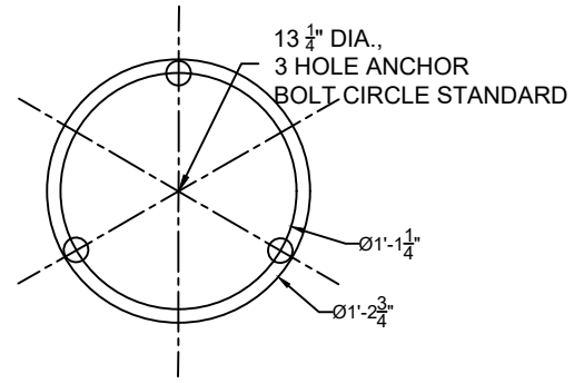
BOLT CIRCLE SCALE: 1" = 1'-0" 2
