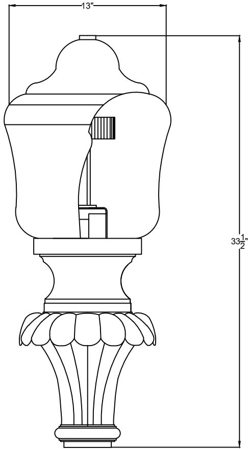
SIDE VIEW SCALE: 1 1/2" = 1'-0"
