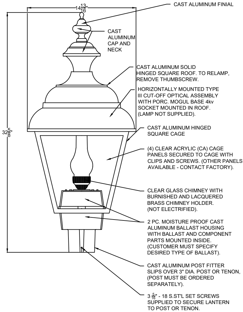
SIDE VIEW SCALE: 1 1/2" = 1'-0"
