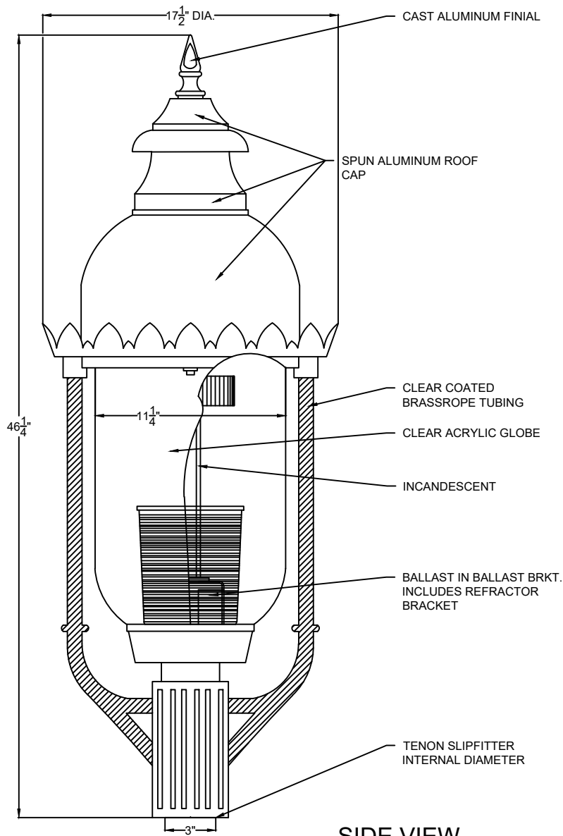
SIDE VIEW SCALE: 1 1/2" = 1'-0"
